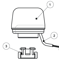
1) Electrothermic actuator 2) Electric cable 3) Thread nut
