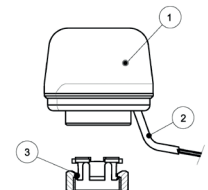
1) Attuatore elettrotermico 2) Cavo elettrico 3) Aggancio rapido
